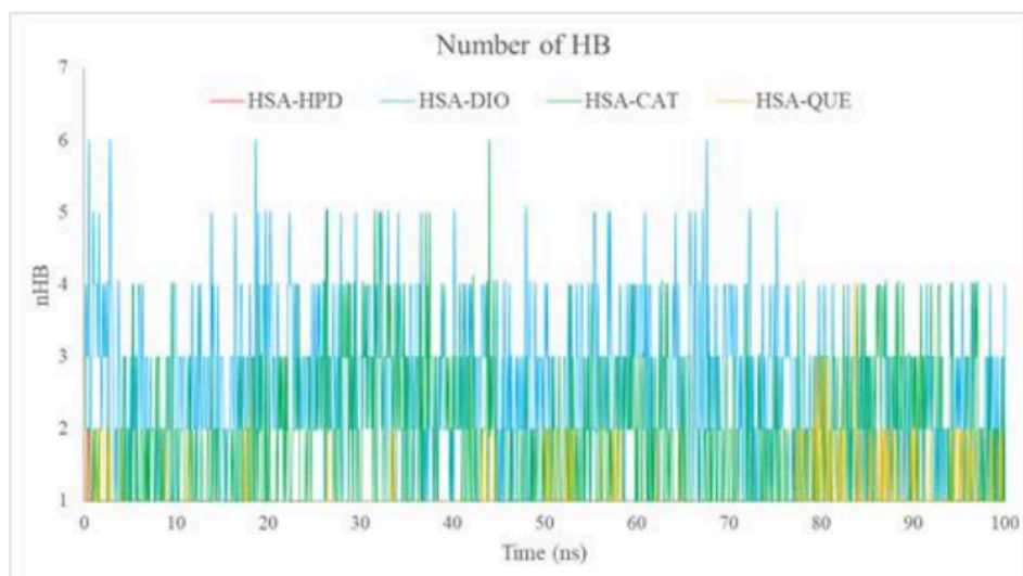
Слика 31. Број водоничних веза (nHB) формираних између HSA и лиганда (HPD, QUE, CAT и DIO) током 100 ns MD симулација.
