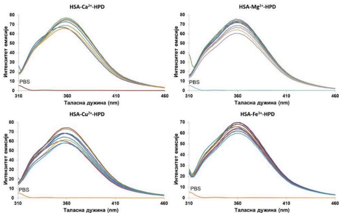
Слика 20. Емисиони спектри HSA-HPD у присуству \text{Ca}^{2+} , \text{Mg}^{2+} , \text{Cu}^{2+} и \text{Fe}^{3+} јона метала ( T = 298 K, \text{pH} = 7,4 ). [\text{HSA}] = [\text{M}^{n+}] 2,0 \mu\text{M} , [\text{HPD}] = 0\text{-}70 \mu\text{M} .
