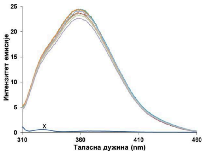
Слика 9. Емисиони спектри HSA у присуству различитих концентрација HPD ( T = 298 \text{ K} , \text{pH} = 7,4 ). [\text{HSA}] = 2,0 \mu\text{M} . Крива x емисиони спектар HPD, [\text{HPD}] = 70 \mu\text{M} .
