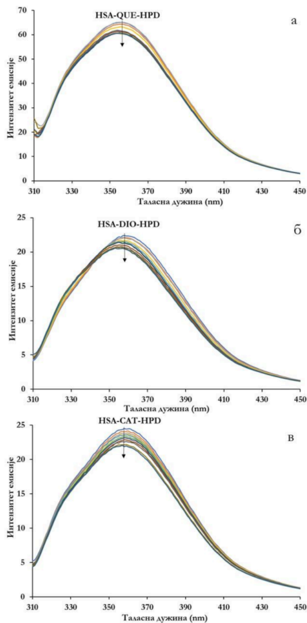
Слика 23. Емисиони спектар HSA-HPD у присуству QUE (а), DIO (б) и CAT (в) ( T=298\text{ K} , \text{pH} = 7,4 ). [\text{HSA}] = 2,0\text{ }\mu\text{M} , [\text{флавоноиди}] = 2,0\text{ }\mu\text{M} и [\text{HPD}] = 0 - 7,05 \times 10^{-5}\text{ M} .
