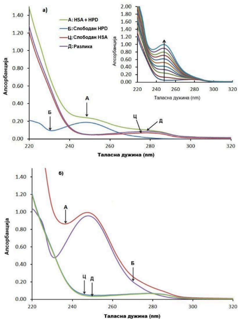
Слика 16. УВ-Вис спектри HSA у присуству HPD: а) апсорпциони спектар HSA-HPD комплекса у односу 1:7 и б) 1:35; А, апсорпциони спектри HSA у присуству HPD; Б, апсорпциони спектар HPD; Ц, апсорпциони спектар HSA; Д, разлика између апсорпционих спектра HSA-HPD комплекса и HPD. На уметнутом делу приказан је апсорпциони спектар HSA у присуству растућих концентрација HPD. [HSA] = 2,0 \mu M , [HPD] = 0 - 70 \mu M .
