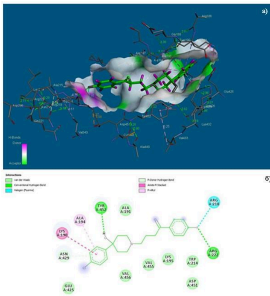
Слика 19. Најдоминантнија конформација халоперидола докованог на албумину (а) основне 2Д HSA-HPD интеракције (б)
