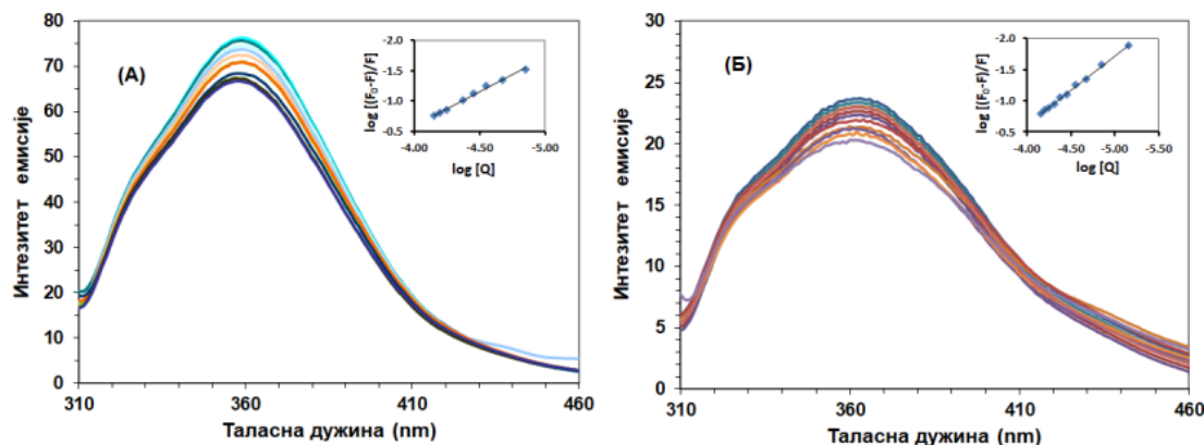
Слика 17. Емисиони спектри HSA-IP (А) и HSA-WF (Б) у присуству различитих концентрација HPD ( T = 298\text{ K} , \text{pH} = 7,4 ). [\text{HSA}] = [\text{IP или WF}] = 2,0\text{ }\mu\text{M} , [\text{HPD}] = 0\text{--}70\text{ }\mu\text{M} . На уметнутом делу је дијаграм логаритамске зависности \log(F_0 - F)/F у односу на \log [Q] .
